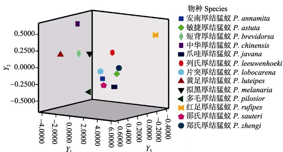
图 1 主成分得分散点图
