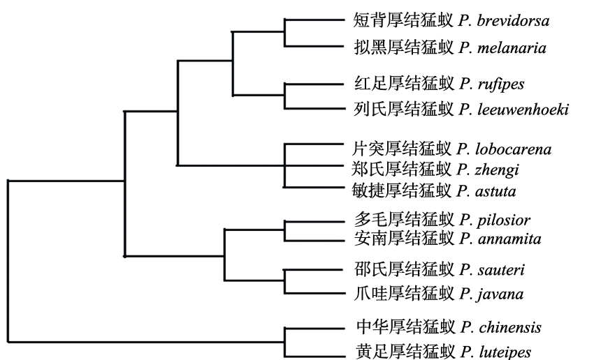
图 2 厚结猛蚁属 13 种蚂蚁系统聚类图
