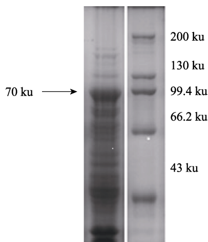
图 1 FPT3 菌株 SDS-PAGE 电泳结果 Fig. 1 SDS-PAGE electrophoresis result of FPT3 strain
