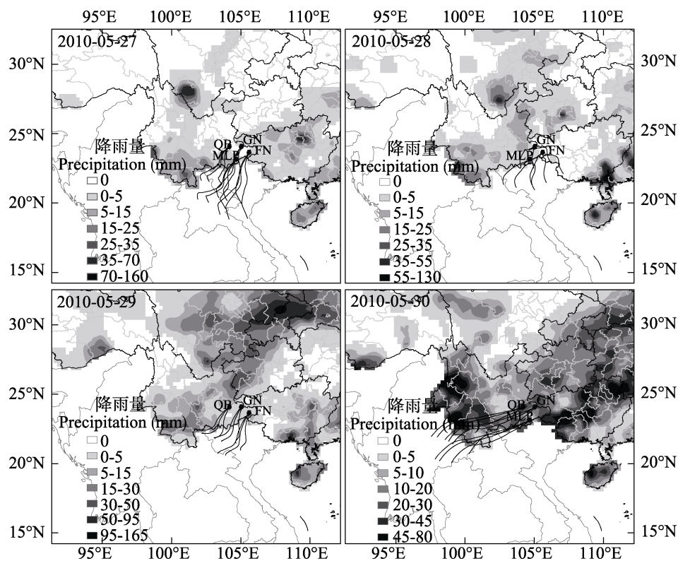
图4 2010年5月27—30日滇东南白背飞虱迁飞路径回推轨迹和累计降雨量
