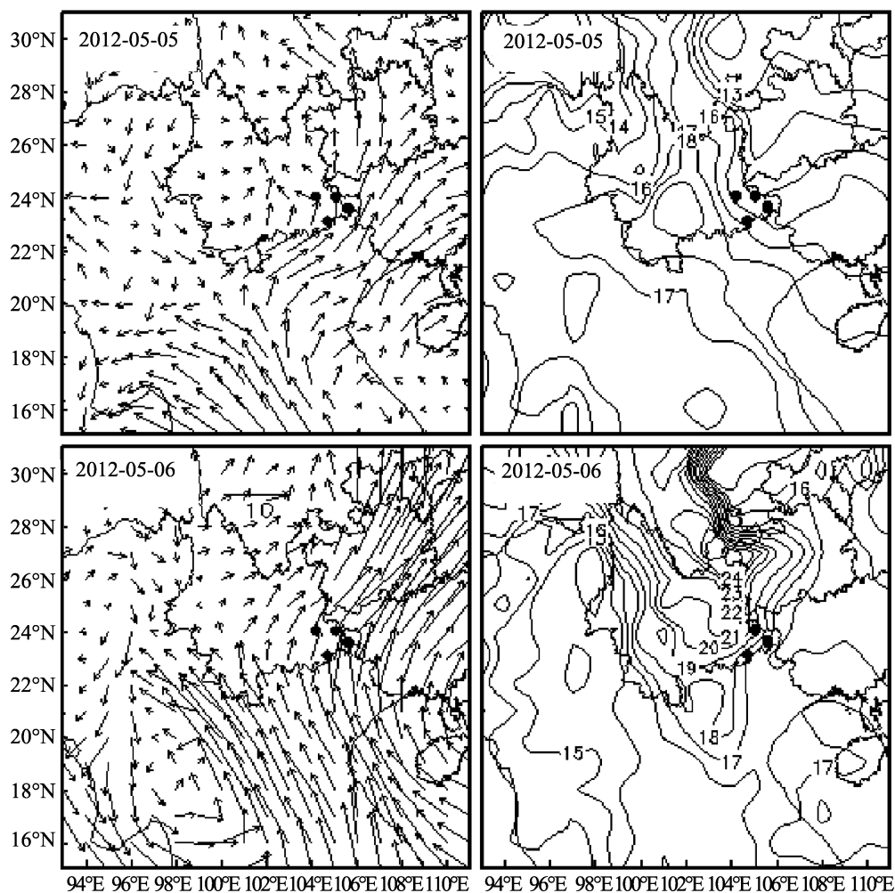
图 11 2012 年 5 月 5—6 日 800 hPa 上的水平风场 (左) 和温度场 (右)
