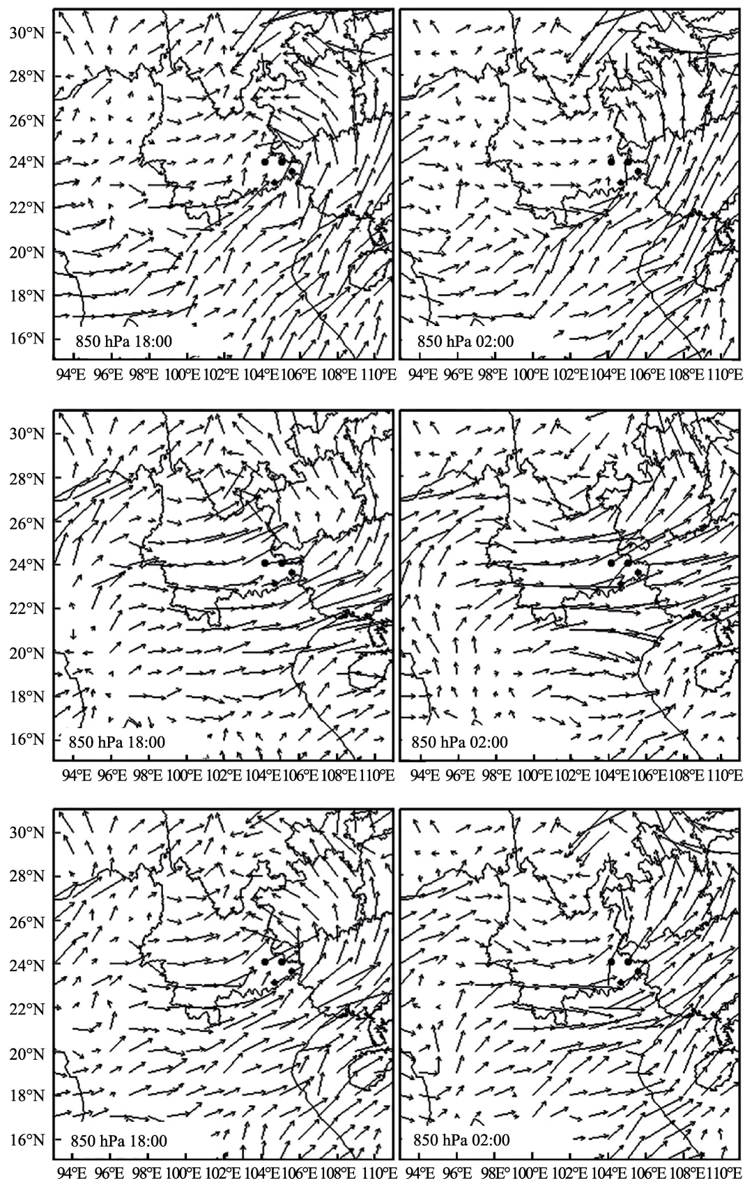
图 14 2010 年 5 月 5 日 850 hPa、800 hPa 和 750 hPa 上的水平风场
