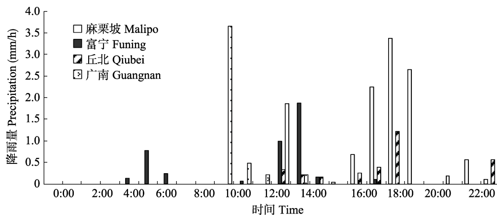
图 7 2010 年 5 月 28 日滇东南富宁、麻栗坡、广南和丘北逐时降雨量 (mm/h) 分布
