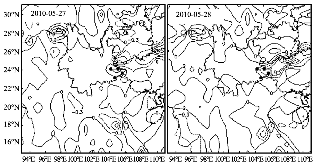
图 5 2010 年 5 月 27 日和 28 日 800 hPa 高度上垂直速度场
