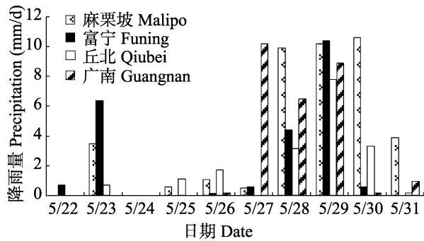
图3 2010年5月22—31日滇东南富宁、麻栗坡、广南和丘北24 h降雨量分布
