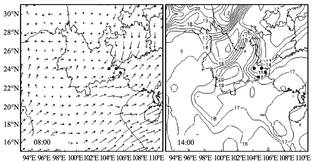
图 6 2010 年 5 月 28 日 800 hPa 高度上水平风场 (左) 和温度场 (右)
