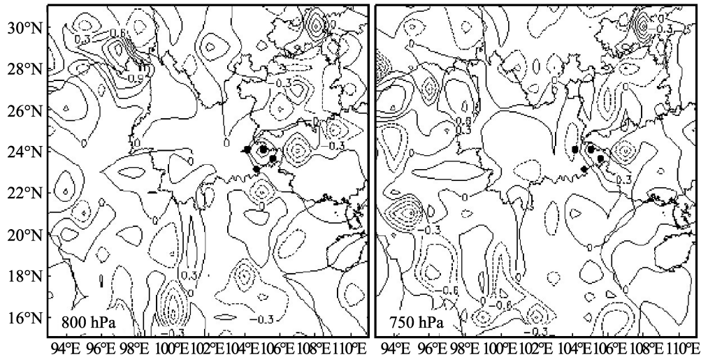
图 12 2012 年 5 月 5 日 800 hPa 和 750 hPa 上垂直速度场 Fig. 12 Vertical velocity (Pa/s) at 800 hPa and 750 hPa on 5 May, 2012
