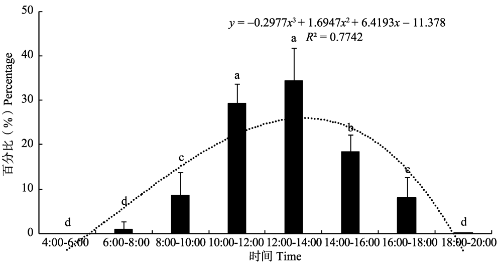
图 2 杏花访花昆虫活动节律 Fig. 2 The activity rhythm of pollinators on apricot flower 柱上标有不同小写字母表示经 Duncan's 多重比较差异显著 (P<0.05)。
