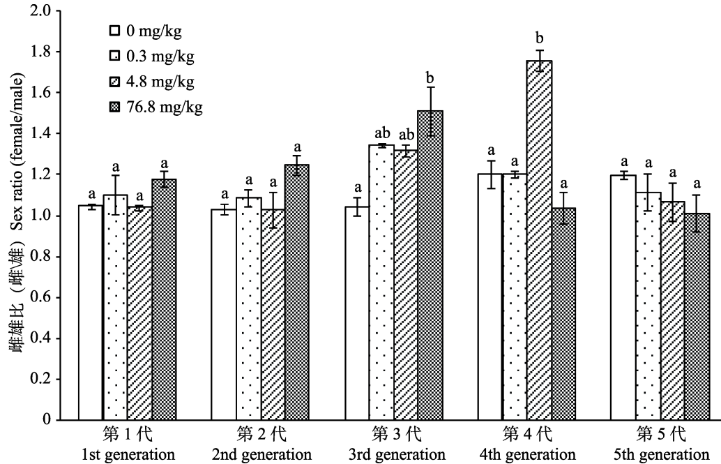
图 1 不同浓度的 Pb^{2+} 胁迫对连续 5 代甜菜夜蛾成虫雌雄比的影响
