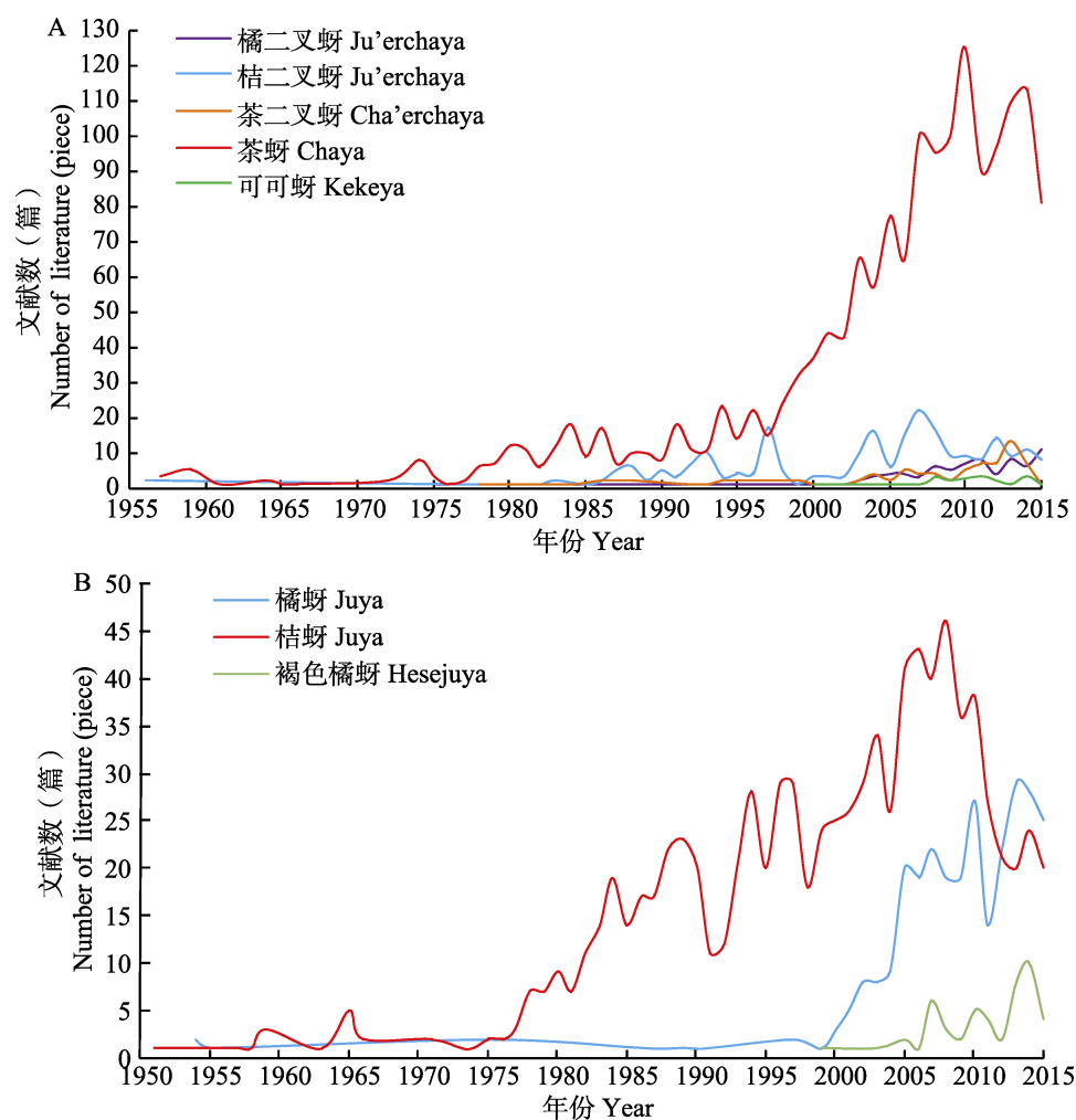
图 2 橘二叉蚜 (A) 和橘蚜 (B) 不同中文名称的使用随时间的变化 Fig. 2 Time-series trends of the usage of different Chinese names of Aphis (Toxoptera) aurantii (A) and A. (T.) citricidus (B) in Chinese scientific papers
