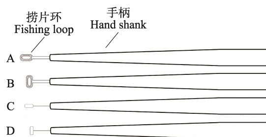
图 5 捞样器示意图
