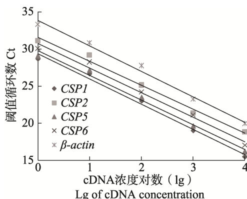
图 4 Amel-CSP1 , Amel-CSP2 , Amel-CSP6 和 \beta -actin 的标准曲线 Fig. 4 Standard curves of Amel-CSP1 , Amel-CSP2 , Amel-CSP6 and \beta -actin
