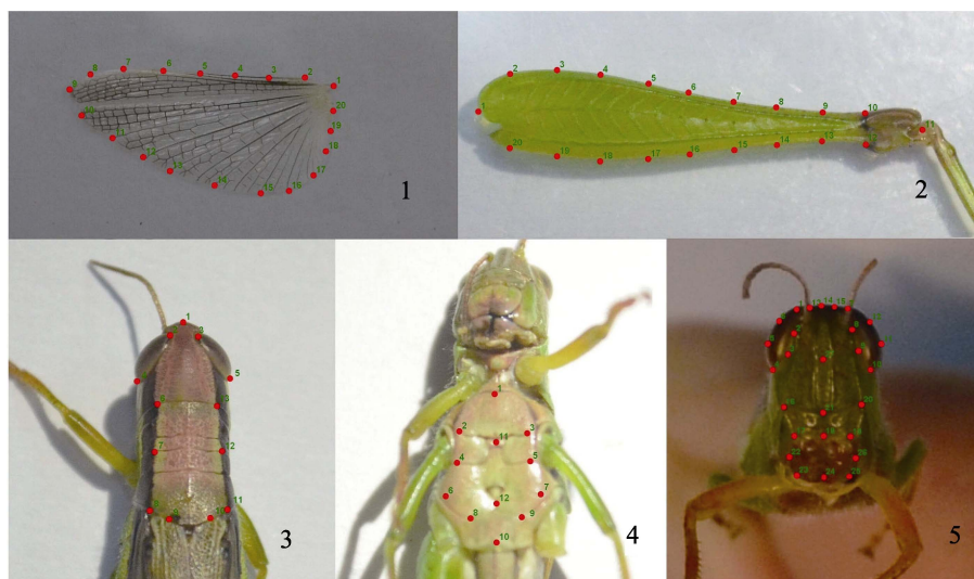
图 1 中华稻蝗的后翅 (1)、后足股节 (2)、前胸背板 (3)、腹板 (4)、颜面 (5) 各结构的地标点
