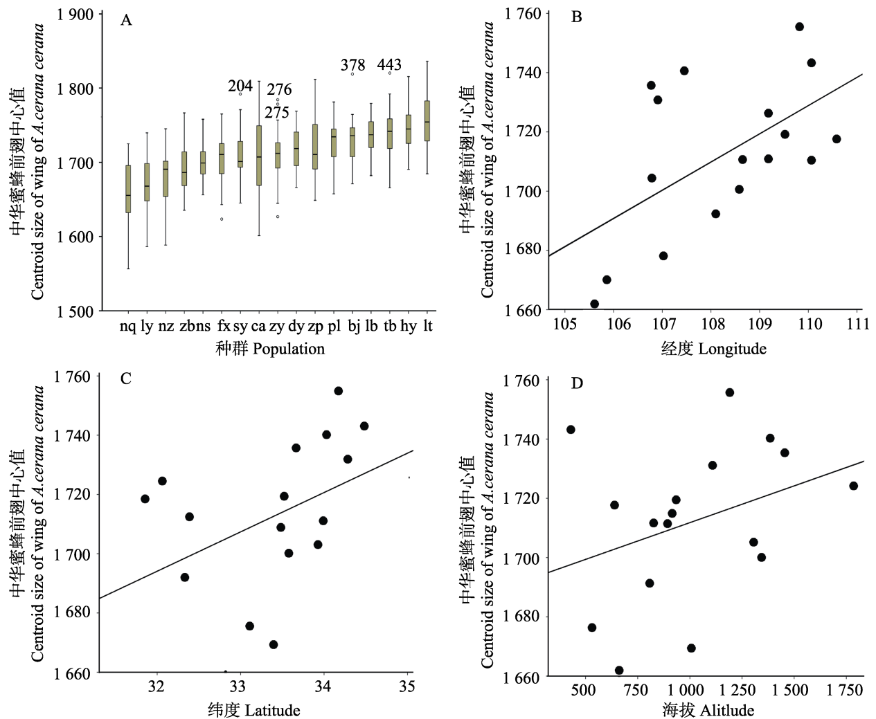
图3 实验中所选 17 个样地翅大小变异图
