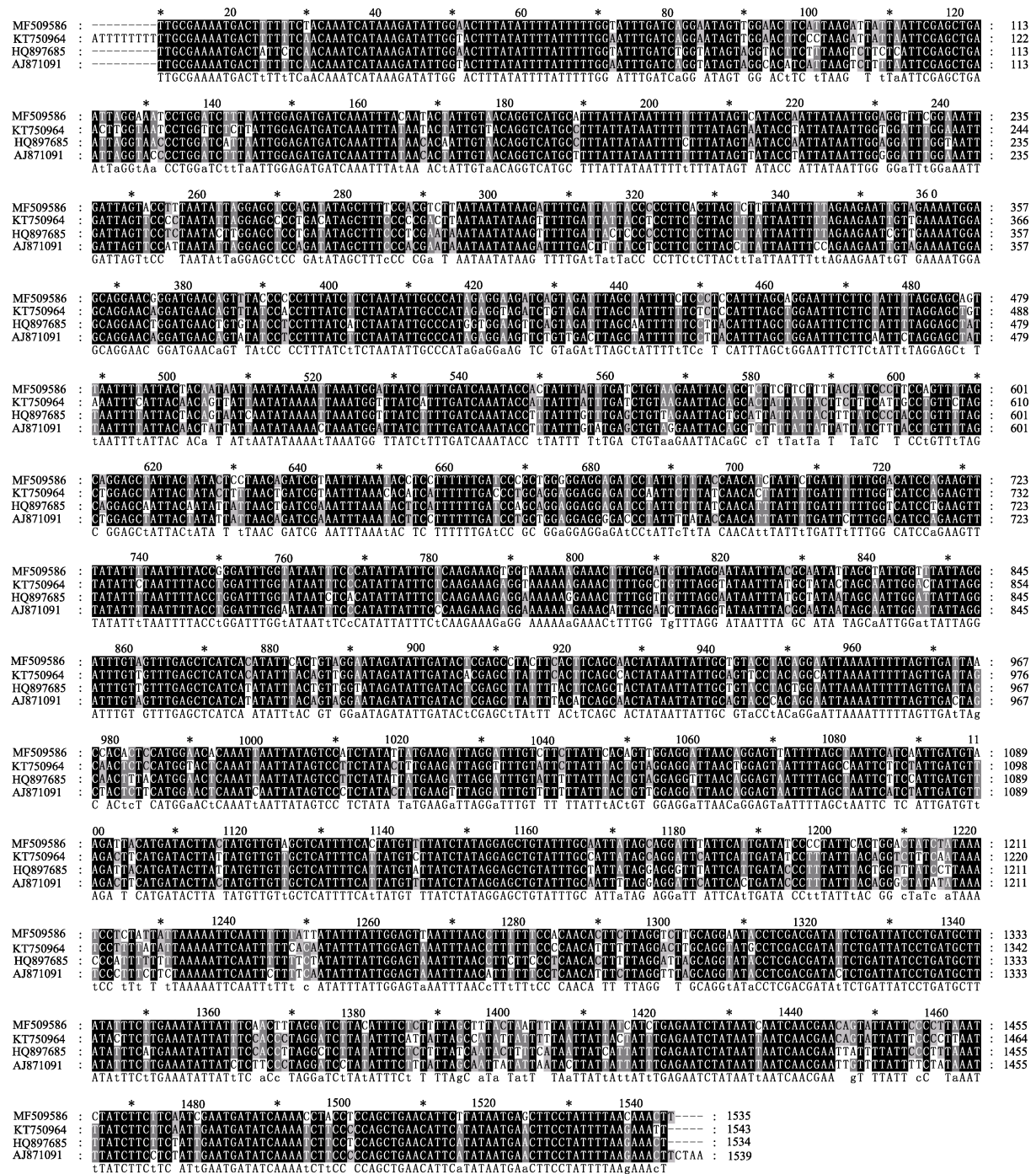
图 2 小蜡螟和其他螟蛾科昆虫 CO I 基因的多序列比对
