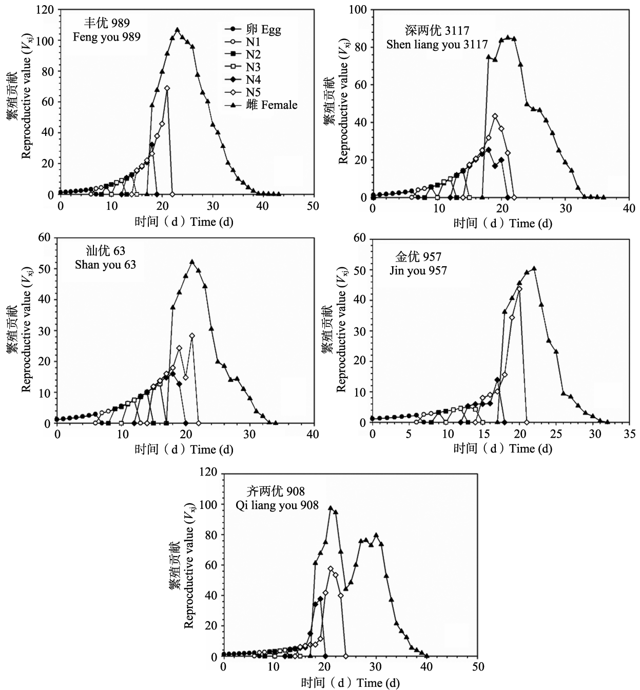
图4 5种水稻品种(“深两优3117”、“金优957”、“齐两优908”、“丰优989”、“汕优63”) 对褐飞虱特定年龄-繁殖贡献( V_{xj} )的影响
