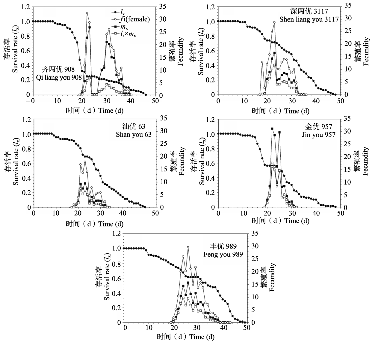
图 5 5 种水稻品种 (“深两优 3117”、“金优 957”、“齐两优 908”、“丰优 989”[lu1]、“汕优 63”) 对褐飞虱特定年龄存活率 ( l_x )、种群年龄特征繁殖力 ( m_x ) 和种群年龄特征净增值率 ( l_x \times m_x ) 的影响
