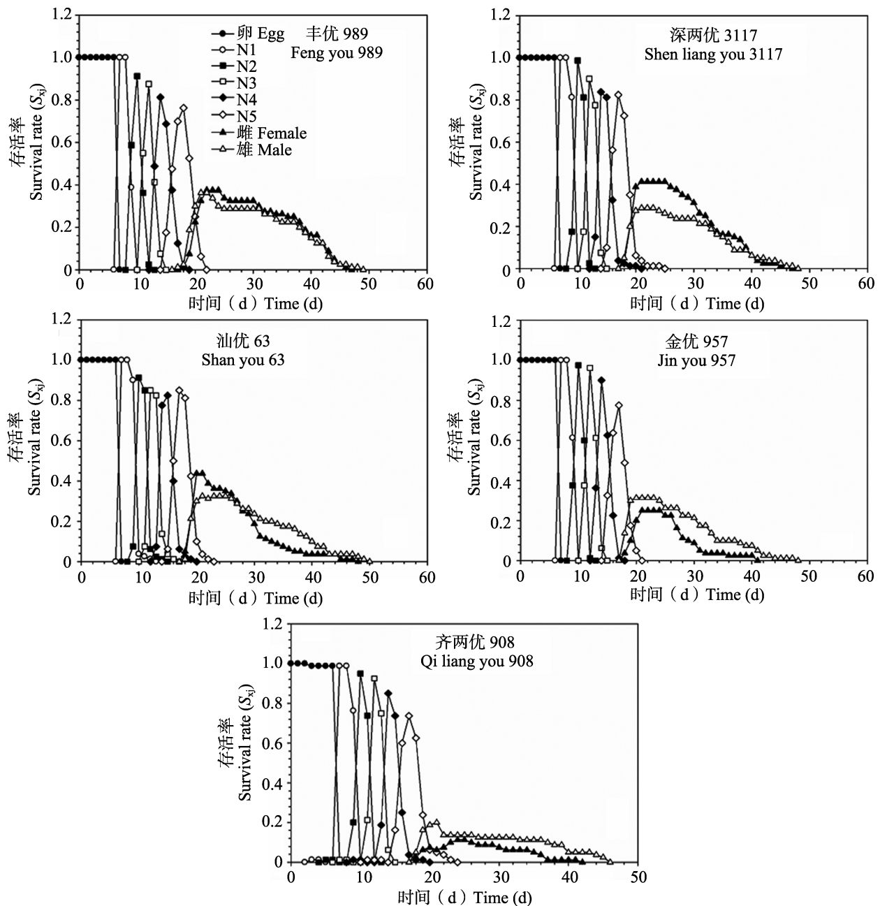
图 3 5 种水稻品种 (“深两优 3117”、“金优 957”、“齐两优 908”、“丰优 989”、“汕优 63”) 对褐飞虱特定年龄龄期存活率 ( S_{xj} ) 的影响
