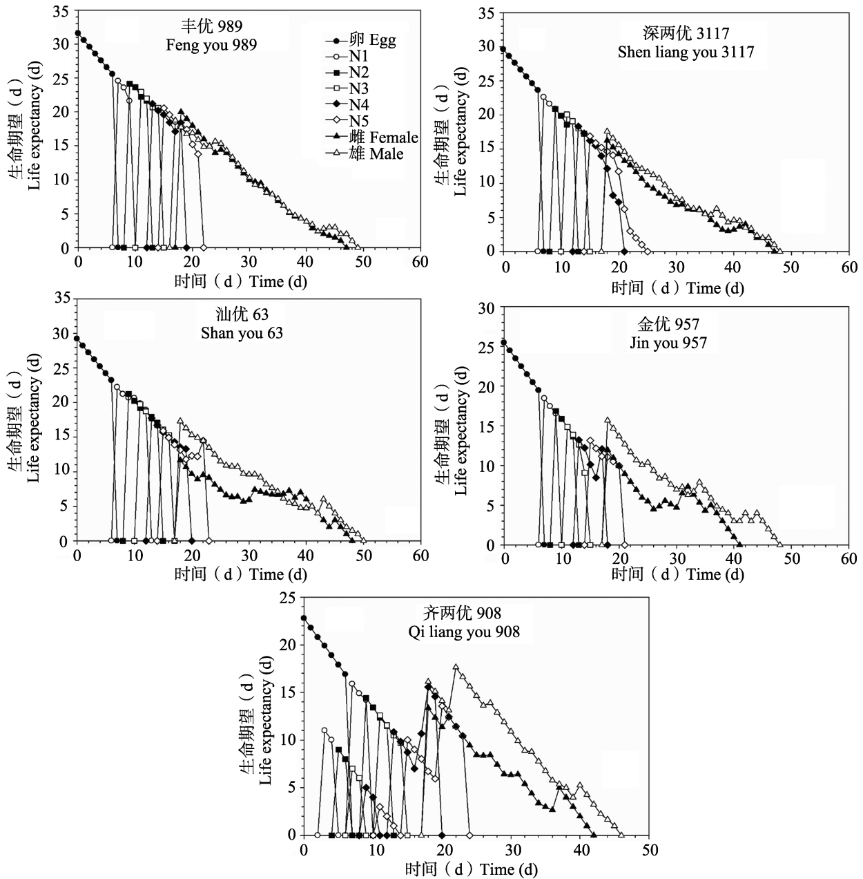
图 1 5 种水稻品种(“深两优 3117”、“金优 957”、“齐两优 908”、“丰优 989”、“汕优 63”)对褐飞虱特定年龄-龄期生命期望( e_{xj} )的影响
