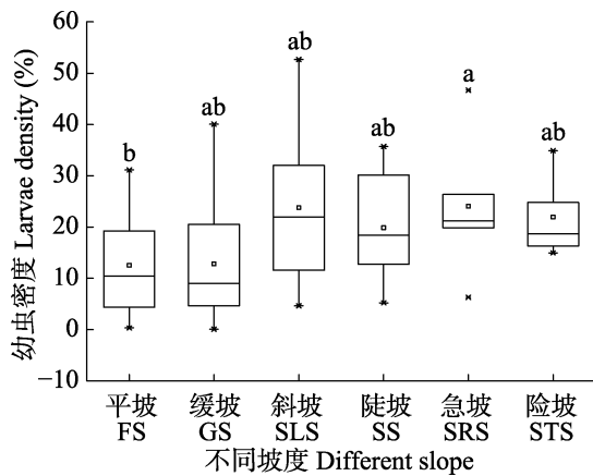
图 6 不同坡度类型榆跳象幼虫密度
