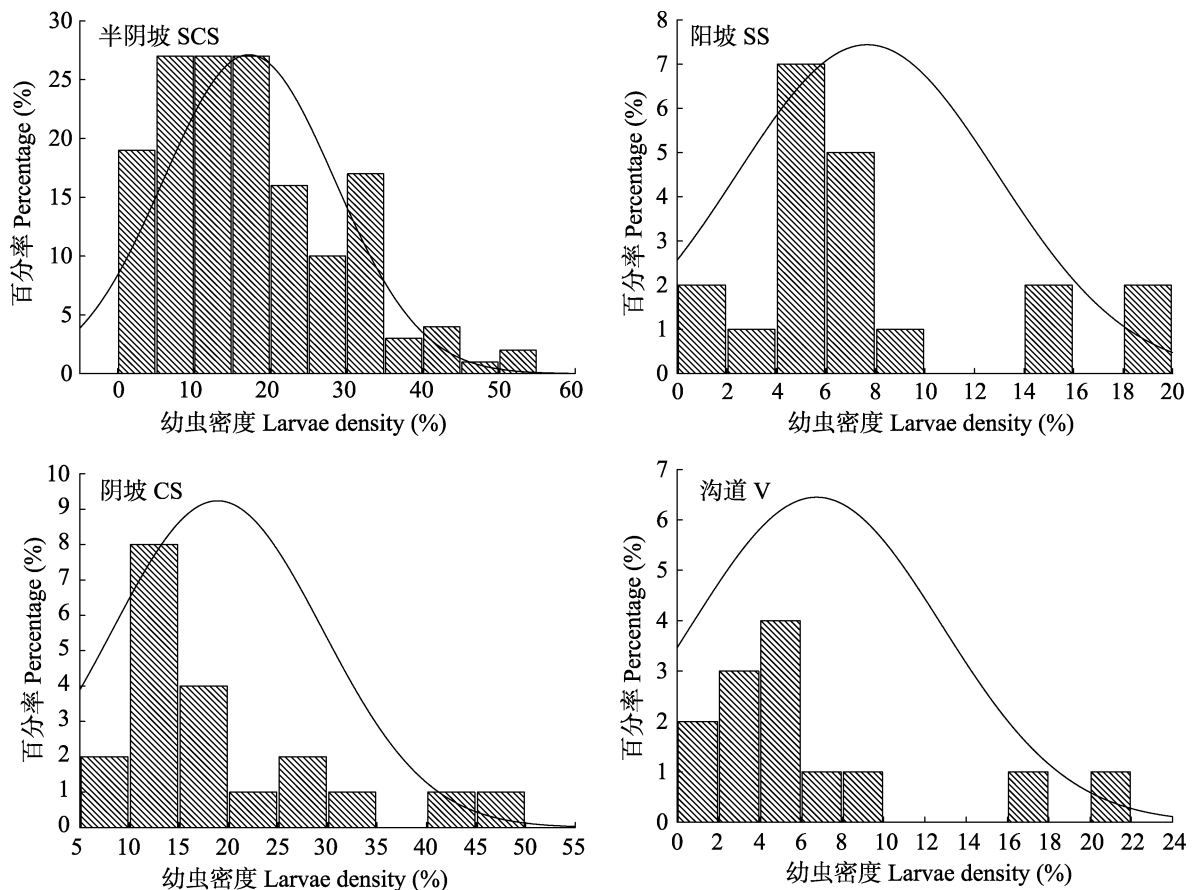
图 1 不同坡向榆跳象幼虫密度分布直方图
