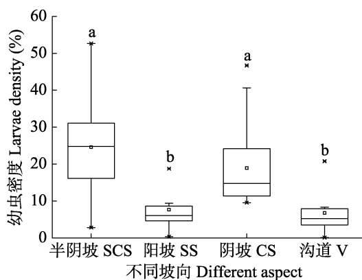
图 2 不同坡向灰榆林榆跳象幼虫密度
