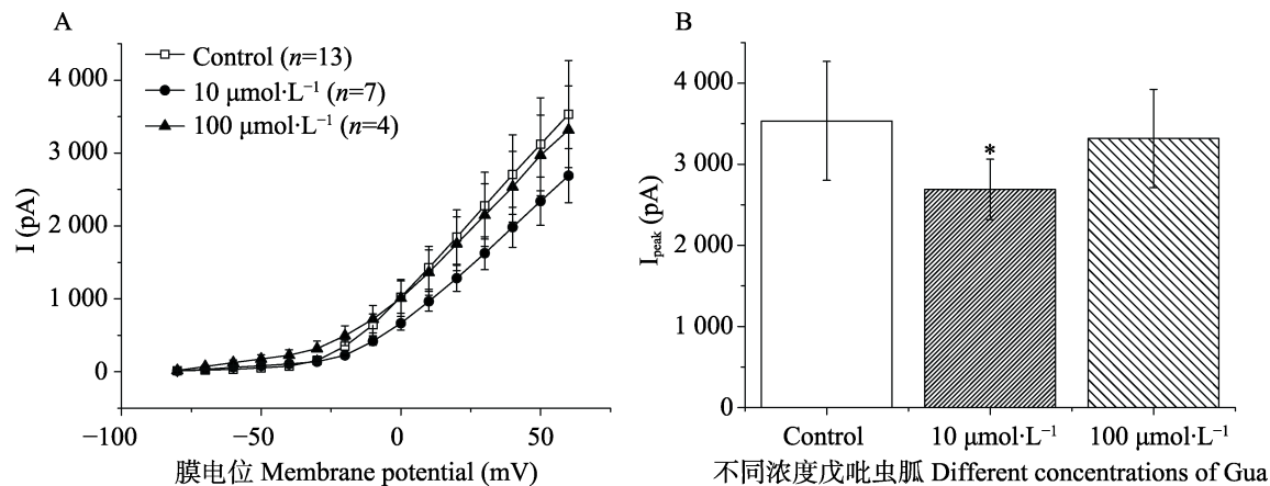
图 7 不同浓度戊吡虫胍作用下 I_K 的 I-V 曲线及 I_{peak} Fig. 7 The I-V curves and I_{peak} of I_K before and after the application of Gua A. 不同浓度戊吡虫胍对棉铃虫中枢神经细胞 K^+ 通道 I-V 曲线的影响: 电流幅值未标准化; B. 戊吡虫胍对棉铃虫中枢神经细胞 K^+ 通道电流的峰值影响。 A. Gua's effects on the I-V curve of K^+ channels: Current amplitude is not standardized; B. The I_{peak} of K^+ channels after Gua.
