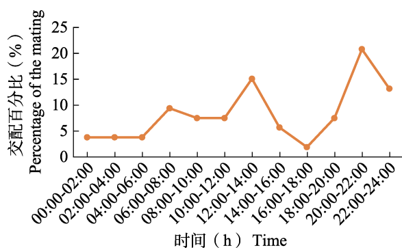
图 4 三叶虫萤交配日节律
