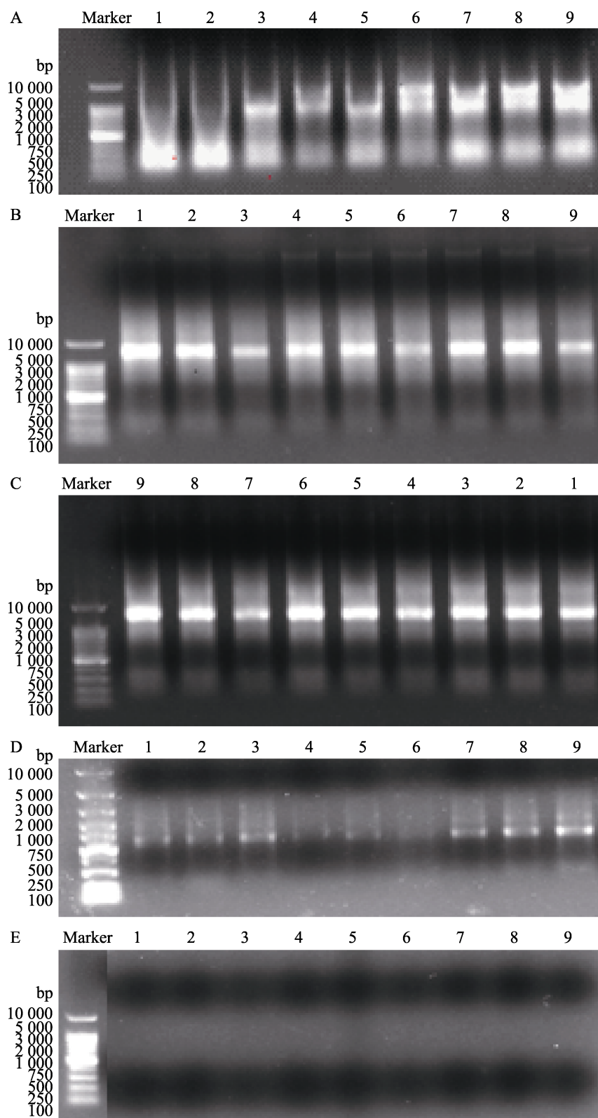
图 2 RNAeasy 动物 RNA 抽提试剂盒琼脂糖凝胶电泳图
