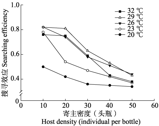
图 2 不同温度下淡足侧沟茧蜂的搜寻效应 与寄主密度的关系
