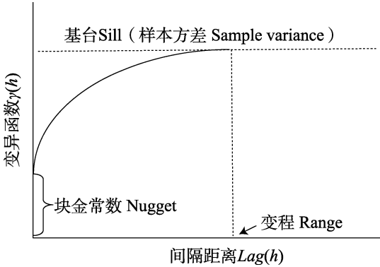
图 1 半变异函数模式图 Fig. 1 A schematic diagram of semivariogram
