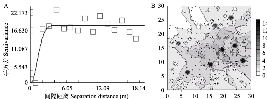
图 6 重度受害林内旧侵入孔数量的半变异函数图 (A) 和等值线与矢量叠加图 (B)
