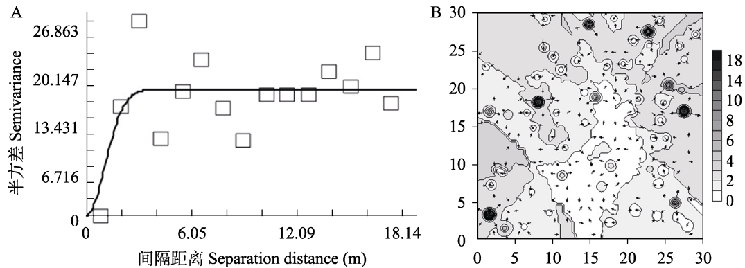
图 5 重度受害林内侵入孔数量的变异函数图 (A) 和等值线与矢量叠加图 (B)
