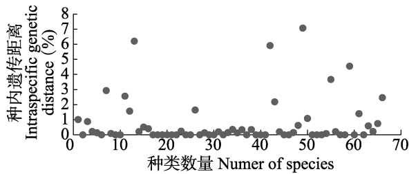
图 3 基于 P 距离 (P-distance) 模型的 28S D2 基因种内遗传距离散点图
