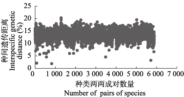
图 2 基于 P 距离 ( P-distance ) 模型的 CO I 基因种间遗传距离散点图 Fig. 2 CO I gene interspecific genetic distances scatter plot based on P-distance model
