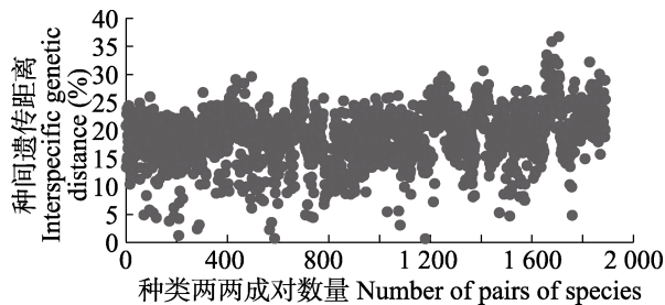
图 4 基于 P 距离 (P-distance) 模型的 28S D2 基因种间遗传距离散点图
