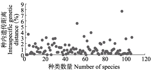
图 1 基于 P 距离 ( P-distance ) 模型的 CO I 基因种内遗传距离散点图 Fig. 1 CO I gene intraspecific genetic distances scatter plot based on P-distance model
