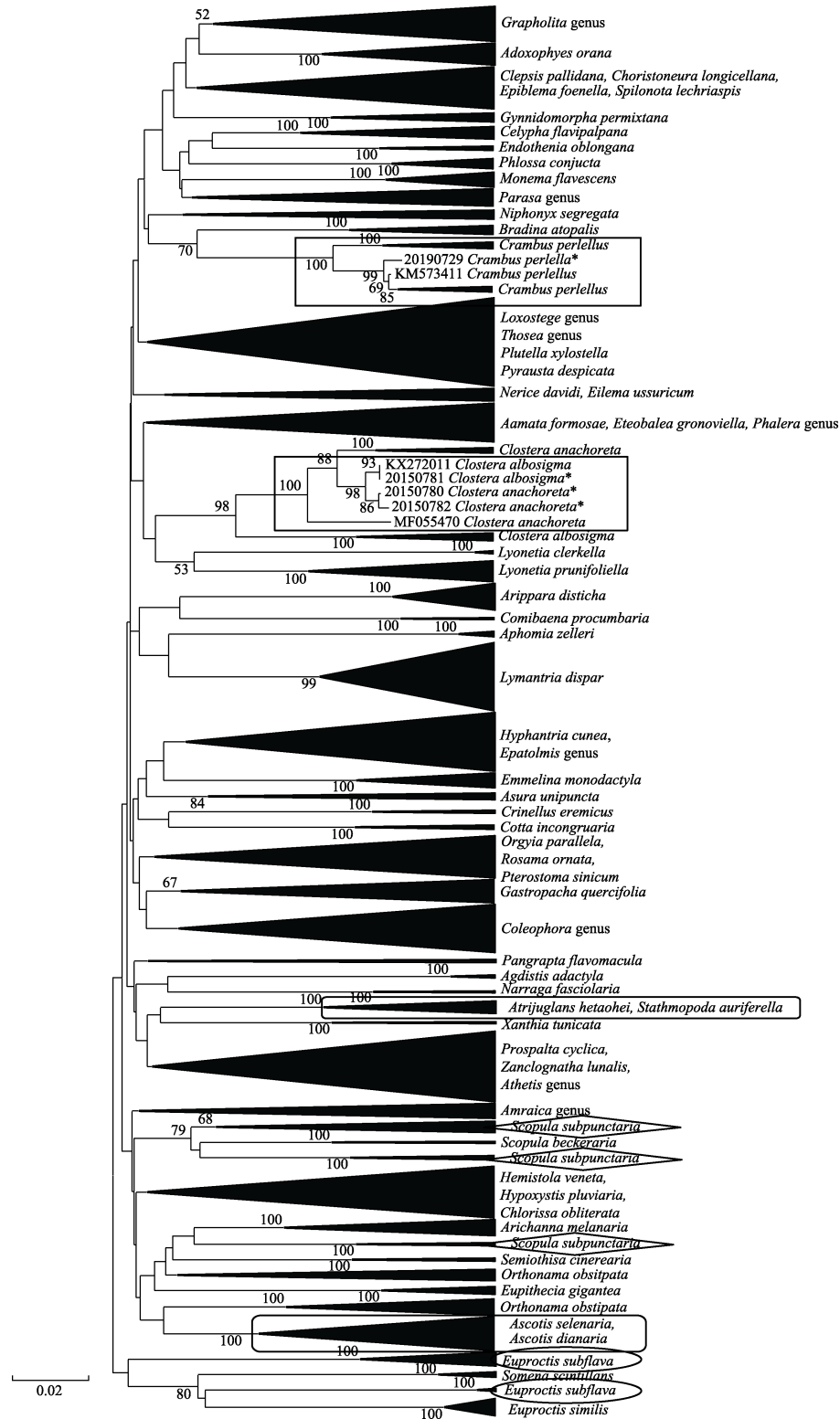
图 5 基于 CO I 基因构建的 NJ 树
