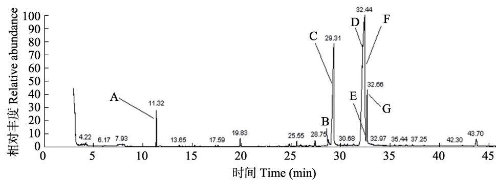
图 1 六星黑点豹蠹蛾雌性信息素腺体提取物 GC-MS 分析的总离子峰图 (TIC) Fig. 1 Mass spectra with EI (70 eV) showing the TIC of sex pheromone gland extracts of Zeuzera leuconotum
