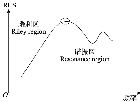
图 2 昆虫 RCS 随频率的响应曲线
