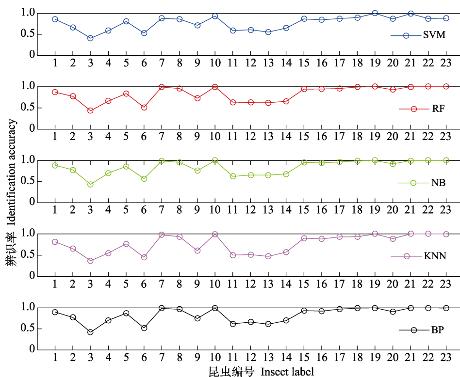
图 5 基于带误差的生物学参数的 23 种昆虫识别率
