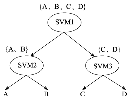
图 3 支持向量机-决策树算法示意图
