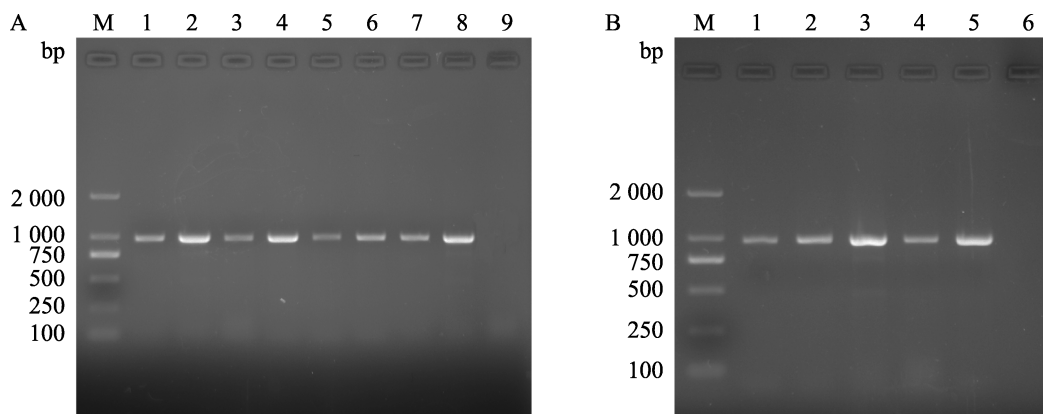
图 1 PCR 检测植物叶片中的 Rickettsia Fig. 1 Rickettsia in plants detected by PCR
