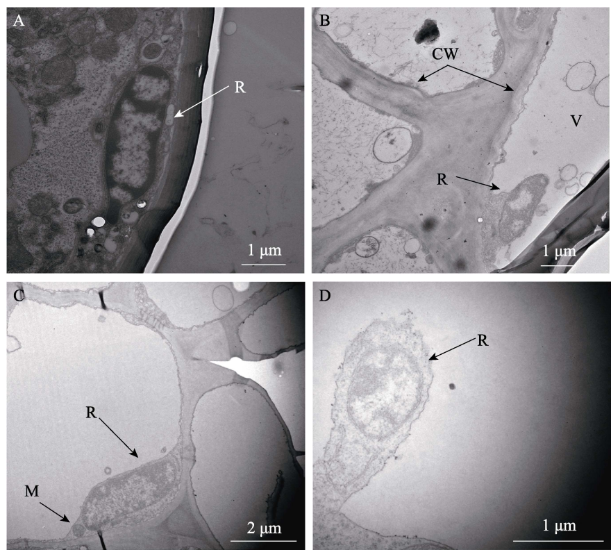
图 2 烟粉虱腹部及植物叶片韧皮部筛管细胞中的 Rickettsia
