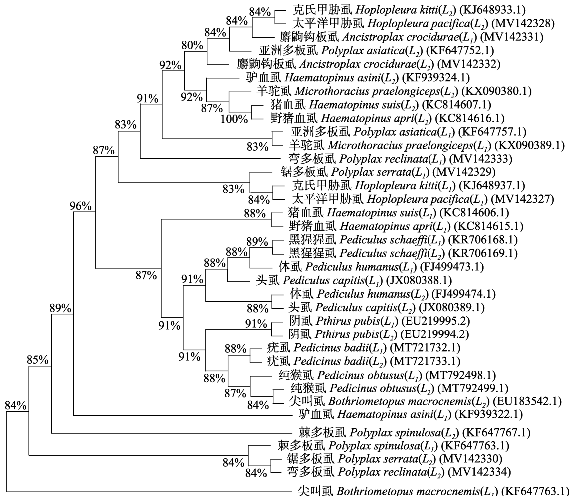
图 4 用 MP 法构建 17 种吸虱 trnL 1 (tag) 和 trnL 2 (taa) 基因序列的进化关系
