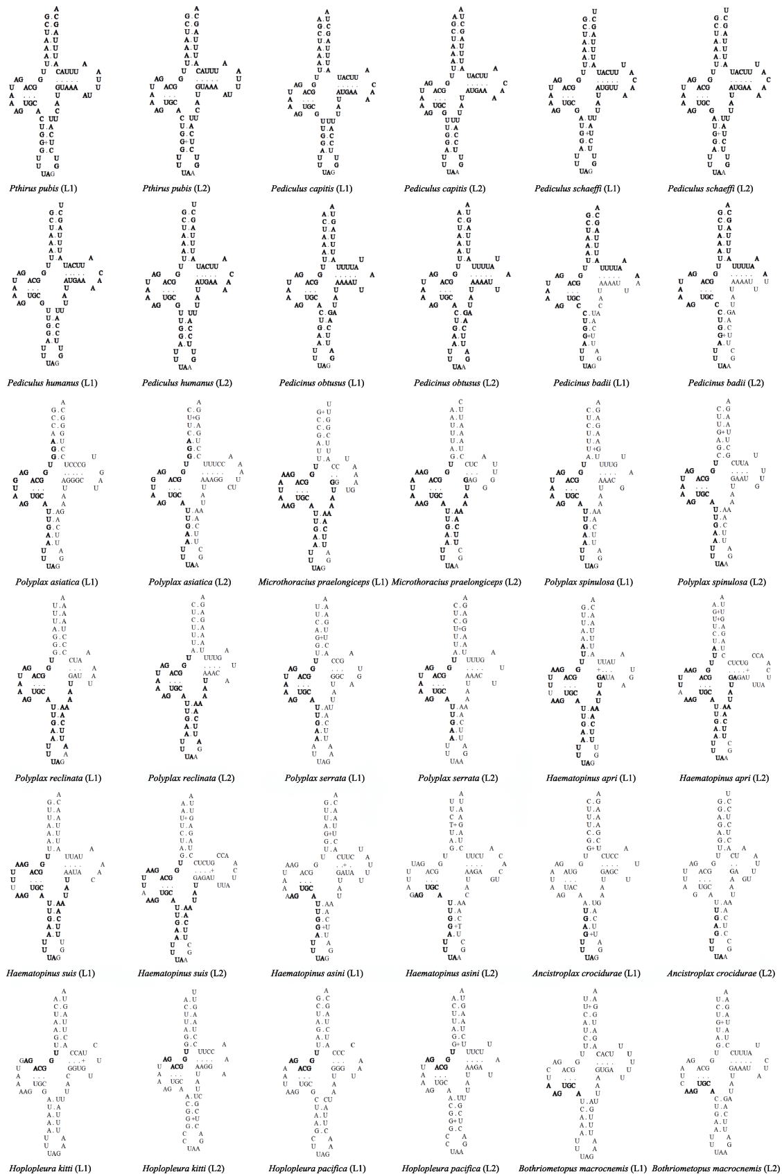
图 1 吸虱和尖叫虱的 trnL 1 (tag) 和 trnL 2 (taa) 基因二级结构图
