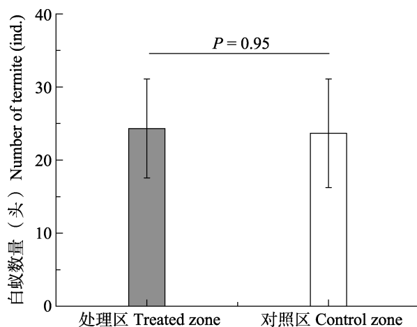
图 2 烯啶虫胺对黑翅土白蚁的驱避作用
