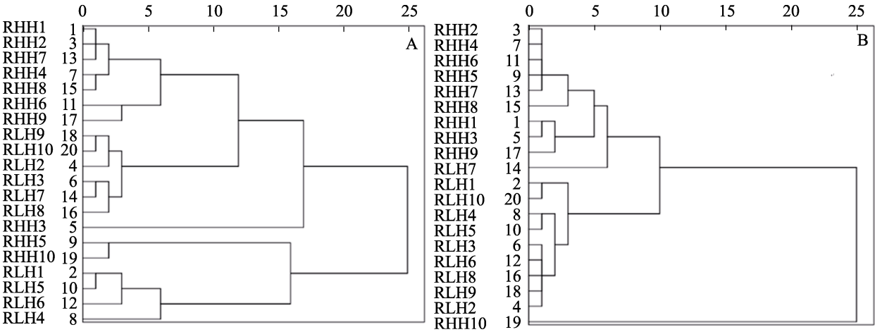
图 1 基于生境异质性分组的群落特征聚类图
