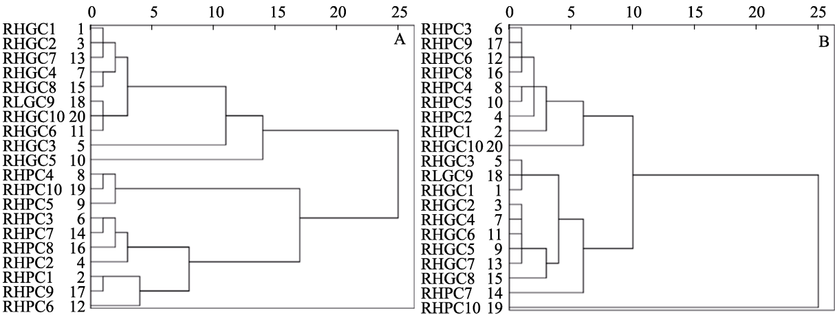
图 2 基于生境连通性分组的群落特征聚类图
