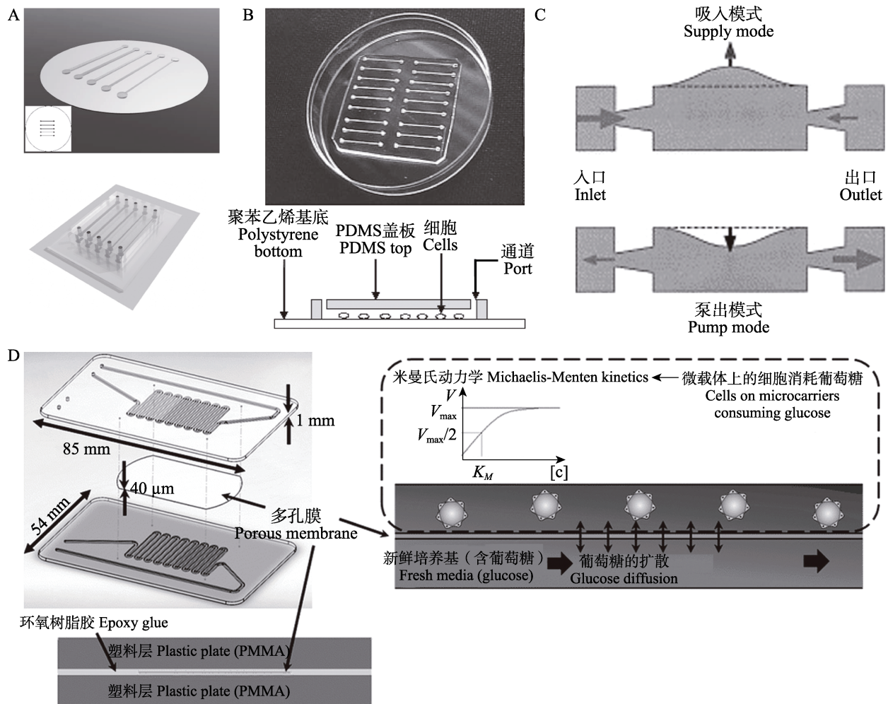
图 1 基于微流控芯片的昆虫细胞系培养
