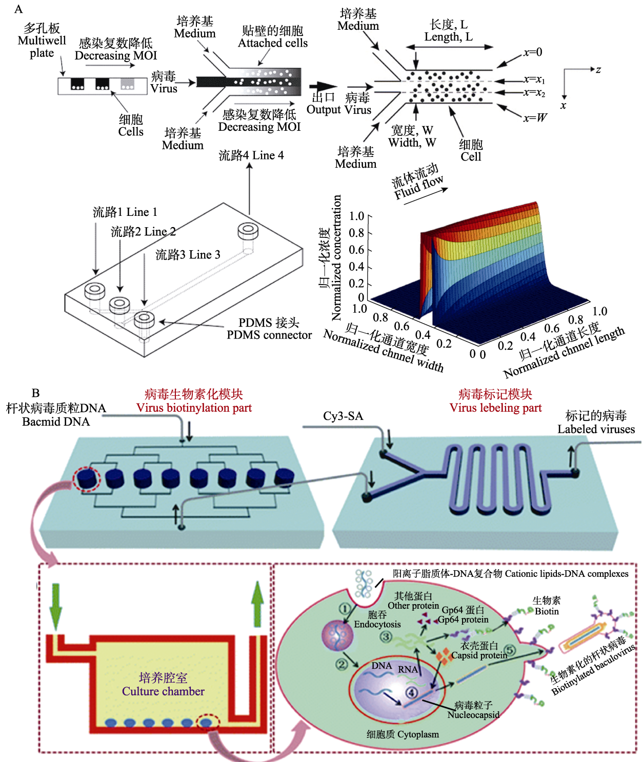
图 4 基于微流控芯片的昆虫病毒研究装置
