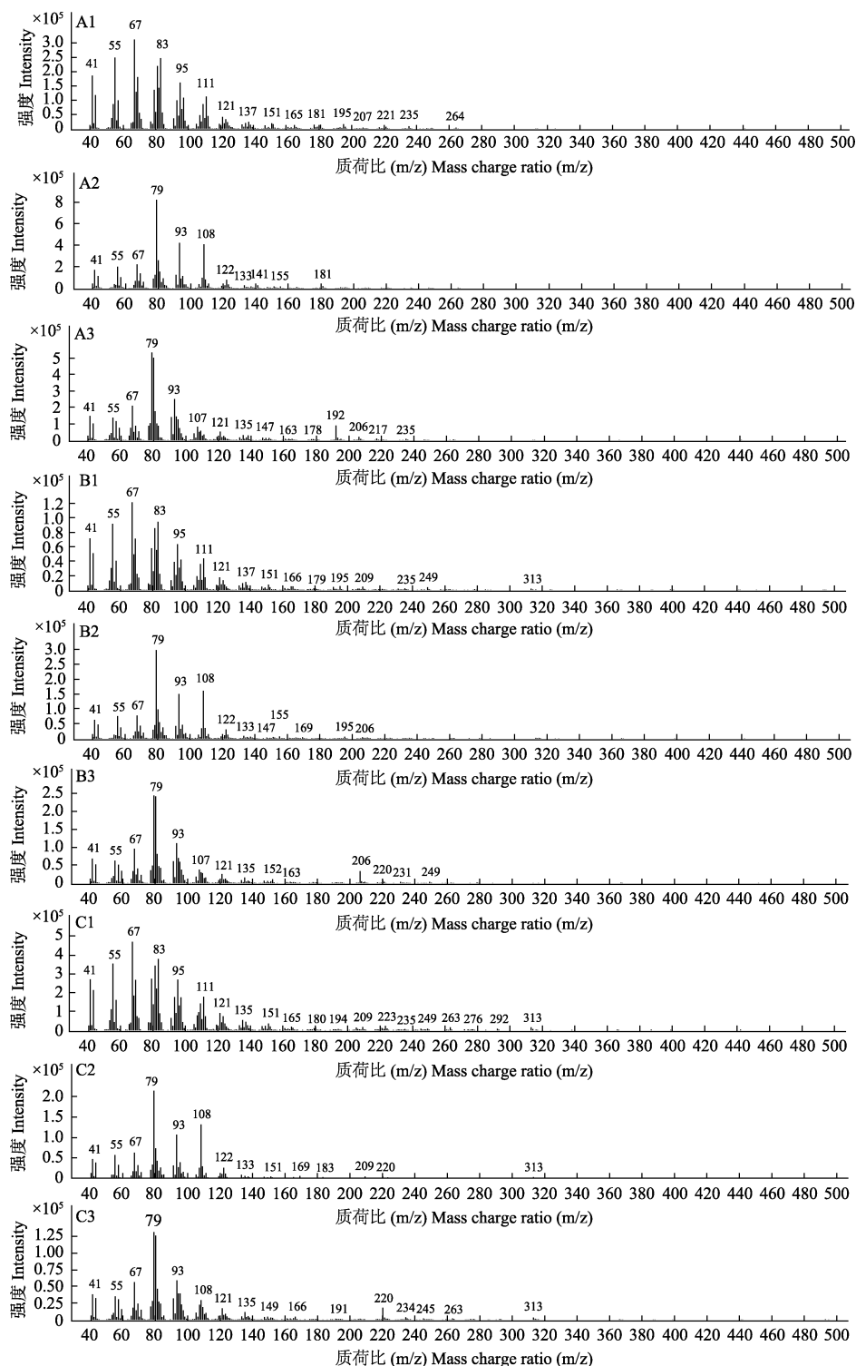
图3 C 18 -C 20 环氧二烯分离制备单体质谱图
