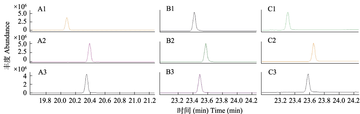
图 2 C_{18} - C_{20} 环氧二烯分离制备单体总离子流图 (TIC)
