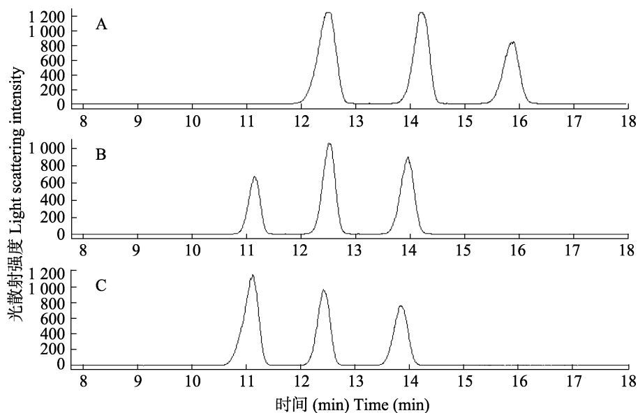
图 1 C_{18} - C_{20} 环氧二烯同分异构体混合分离效果
