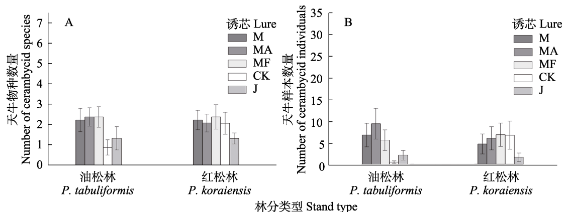
图 5 底物异丙醇 (J) 对广谱型引诱剂 (M) 和复配诱芯 (MA 和 MF) 诱集效果的影响
