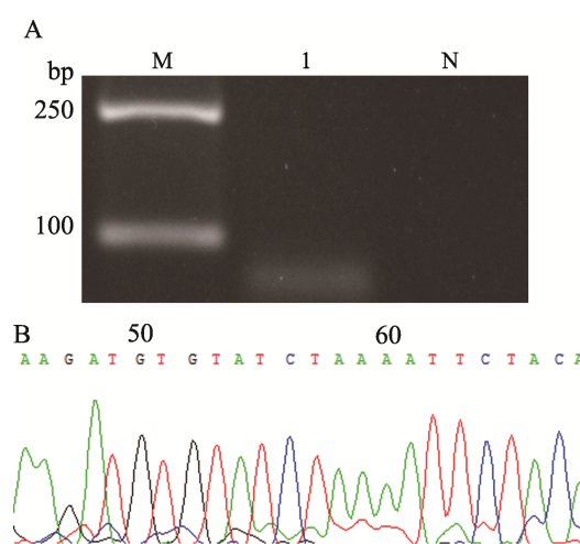
图 1 nce-miR-15325 的 Stem-loop RT-PCR 与 Sanger 测序验证
