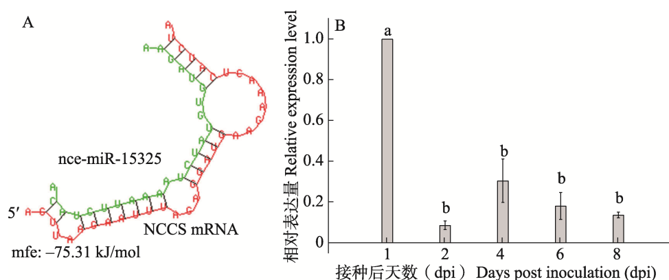
图 4 东方蜜蜂微孢子虫感染意蜂工蜂过程中靶基因 NCCS 的相对表达量检测
