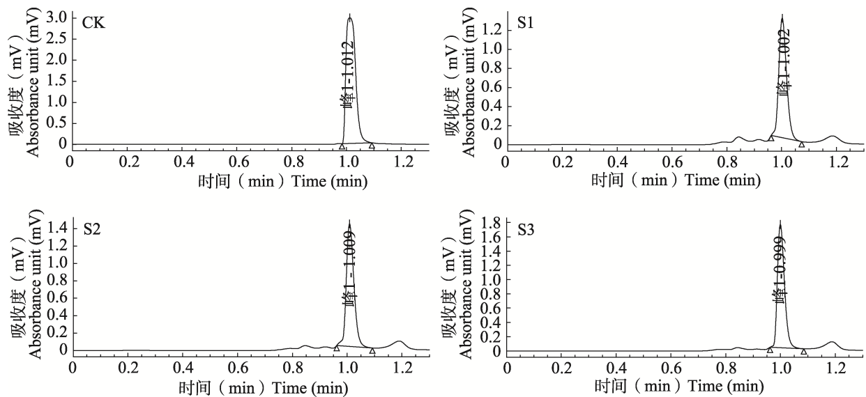
图 4 不同生长阶段腺苷的超高效液相色谱峰图
