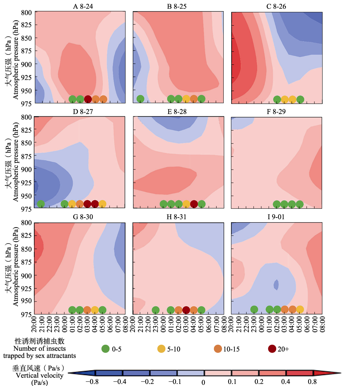
图 5 2021 年稻纵卷叶螟迁飞期间南京 800-975 hPa 20:00-8:00 垂直风速
