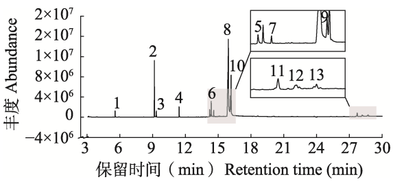
图 1 大斑芫菁浸提物 GC-MS 总离子流色谱图 Fig. 1 GC-MS total ion flow chromatogram of Mylabris phalerata extracts
