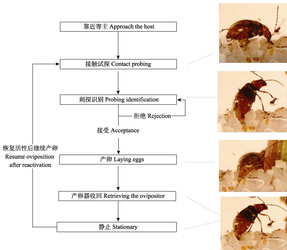
图4 双斑长跗萤叶甲产卵过程
