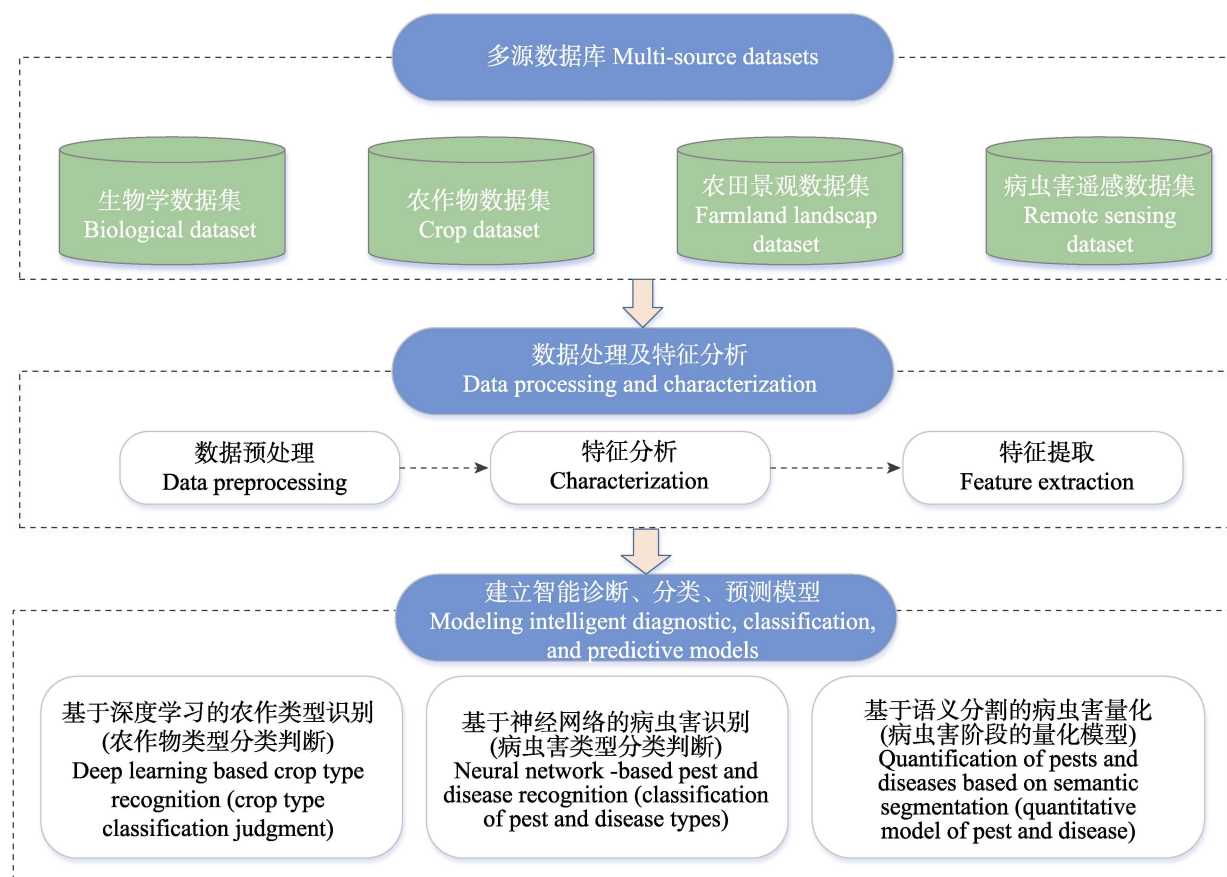
图 2 基于 AI 技术的多源数据驱动的病虫害智能识别与分类建模流程图
