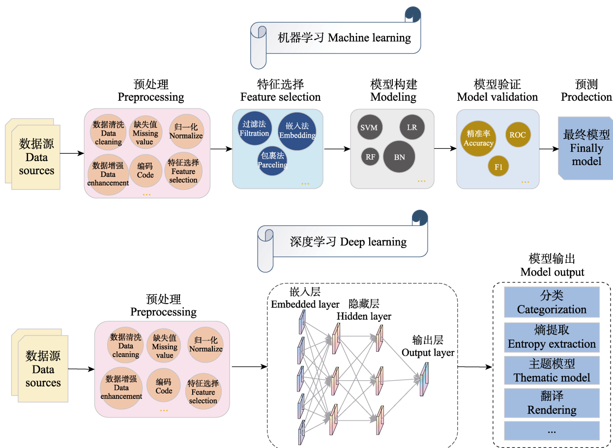
图 1 机器学习和深度学习在建模流程中的理论框架示意图
