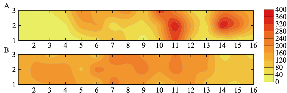
图 3 2023 ( A ) 和 2024 年 ( B ) 田间双斑长跗萤叶甲成虫分布等值线图 Fig. 3 The isogram of Monolepta hieroglyphic adults distribution in the field in 2023 (A) and 2024 (B)
