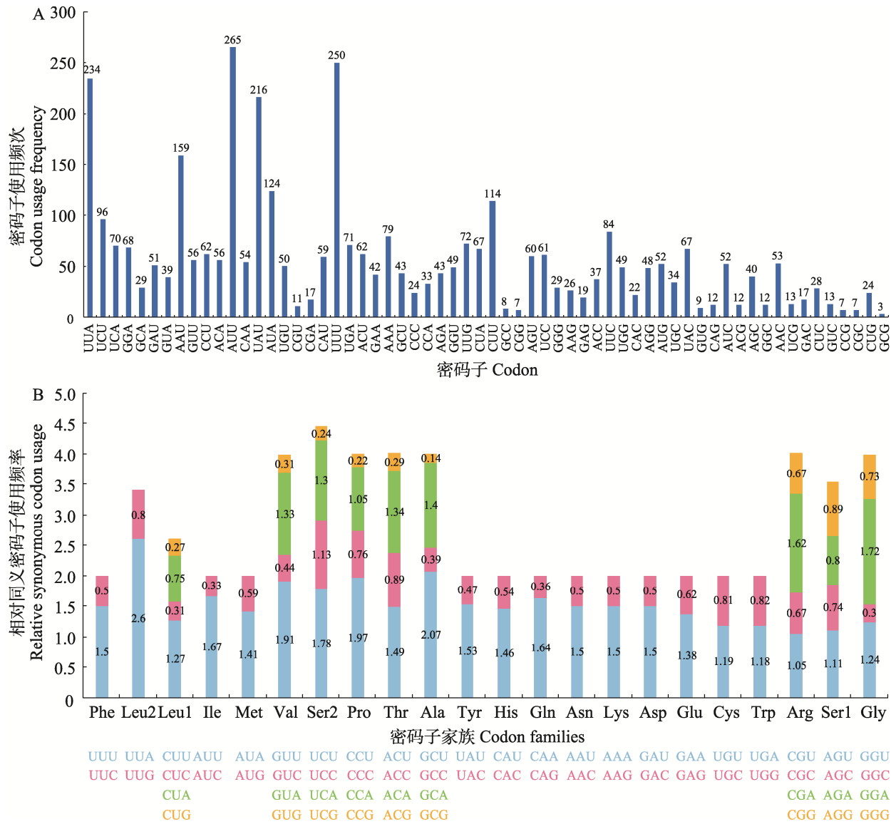
图 2 双带麻蠡线粒体基因组蛋白质编码基因的密码子使用
