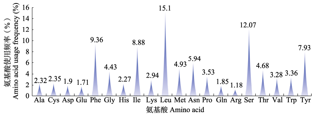
图 3 双带麻蠡线粒体基因组氨基酸组成百分比
