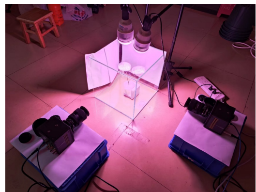
图 2 突眼实蝇起飞实验观测系统的组成及布局
