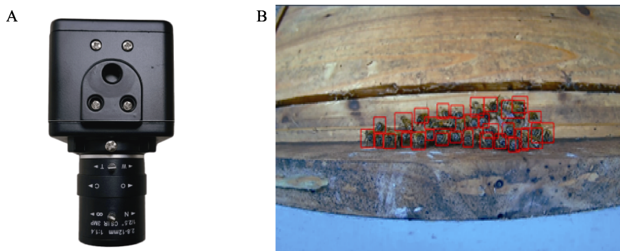
图 5 摄像头 Fig. 5 Camera
