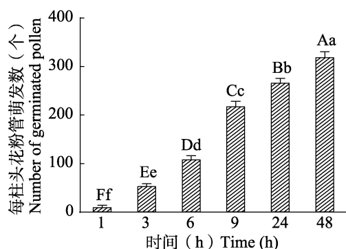
图 2 授粉后不同时间段日光温室番茄 每柱头花粉管萌发数量
