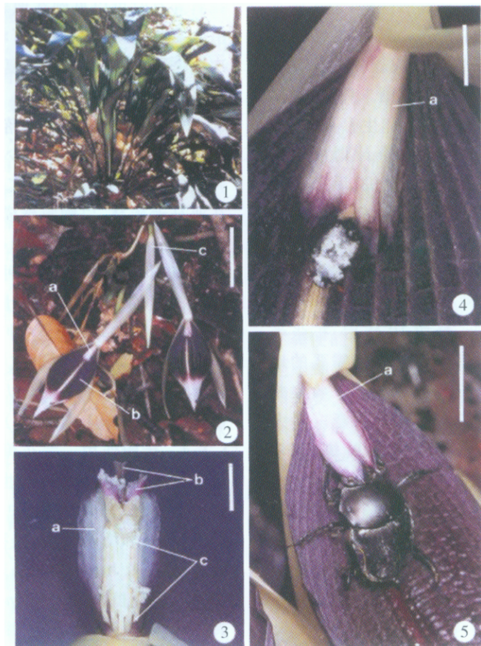
图 1~5 蜣螂的传粉作用(仿 Sakai & Inoue, 1999)
