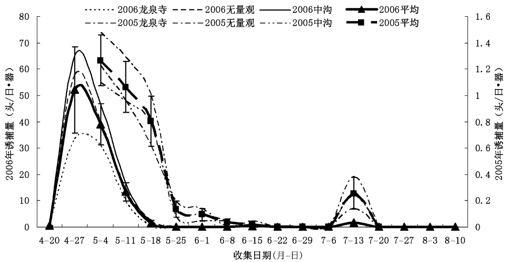
图 3 2005~2006 年横坑切梢小蠹扬飞曲线
