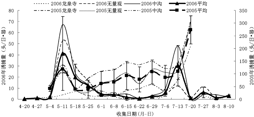
图 1 2005 ~ 2006年黄色梢小蠹扬飞曲线
