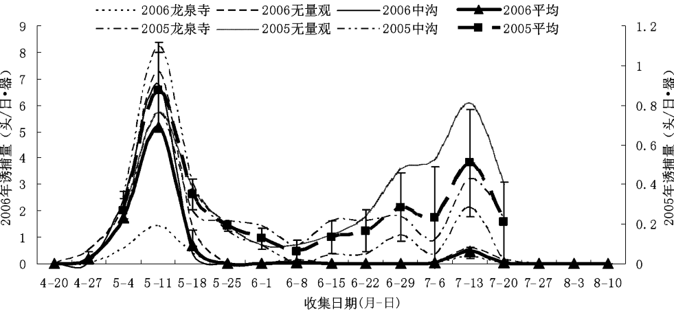
图 2 2005 ~ 2006年红松根小蠹扬飞曲线
