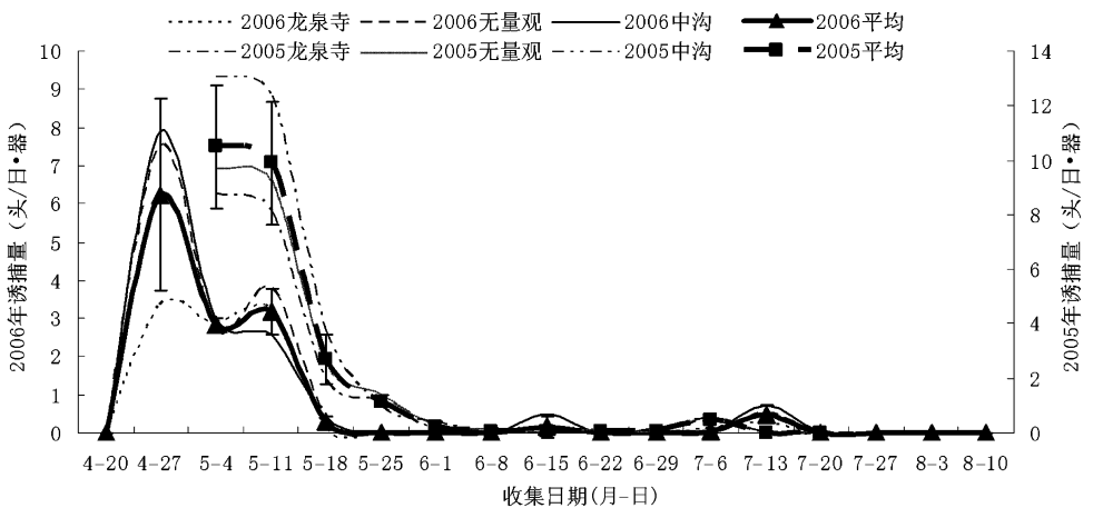
图 4 2005~2006 年纵坑切梢小蠹扬飞曲线
